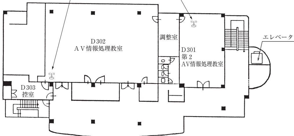
D棟 3F
